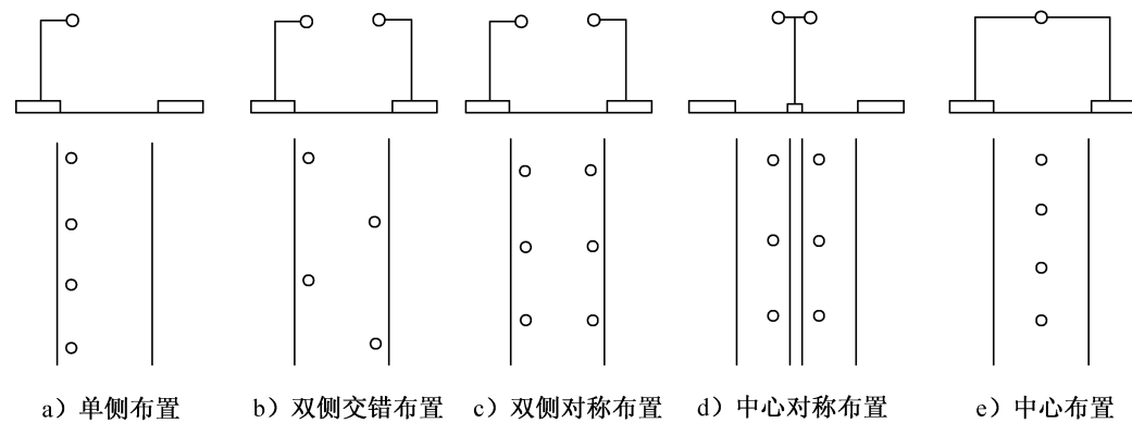
图 1 公路照明布设方式
